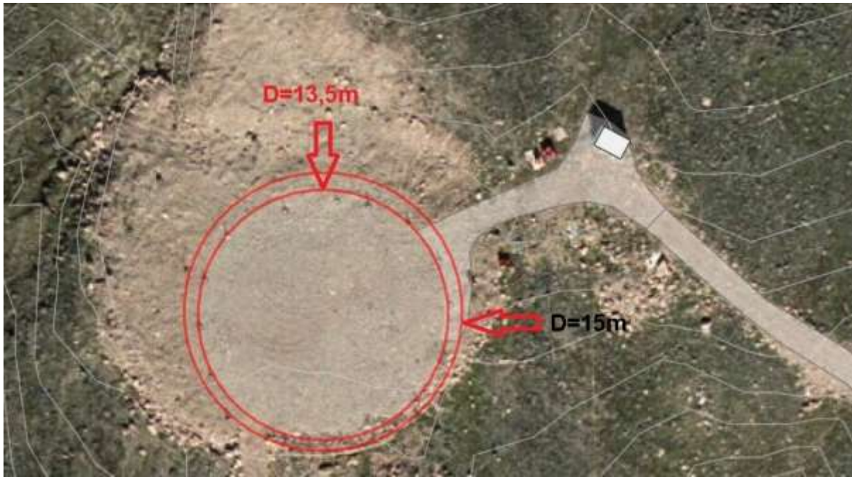
Ilusiliaq 66: Siorapalummi qulimiguulinnut mittarfik (najoqqutarisaq: NunaGis)
