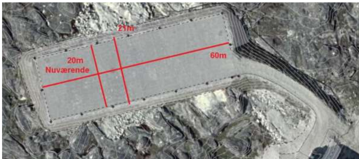
Ilusiliaq 19: Alluitsup Paani qulimiguulinnut mittarfik (najoqqutarisaq: NunaGIS)
