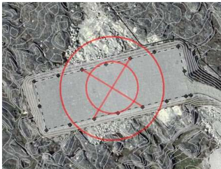
Ilusiliaq 20: Alluitsup Paa (20 x 60m-inik annertussuseqarluni kipparissuusimagaluarluni ammalortumut tukimut 18m-imik annertussusilimmut allanngortinneqarpoq)
