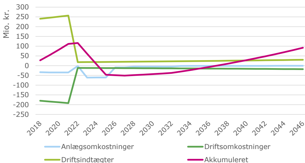
Ilusiliaq 8: Periarfissatut ilusiliaq 5-imut sanaartornermut aningaasartuutit, ingerlatsinermut aningaasartuutit, ingerlatsinermi isertitat kiisalu ingerlatsinerup inerneru tamarmiusoq
