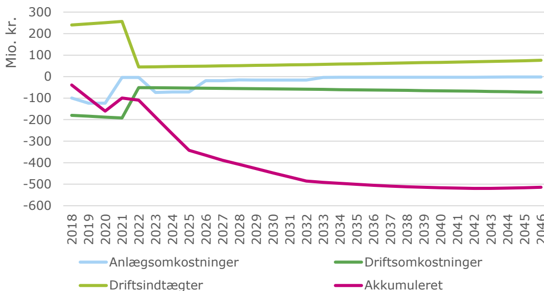
Ilusiliaq 4: Periarfissatut ilusiliaq 1-imit sanaartornermut aningaasartuutit, ingerlatsineranut aningaasartuutit, ingerlatsinermit isertitat kiisalu ingerlatsinerup inernerat tamarmiusoq
